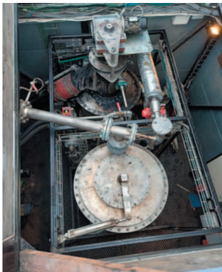
Förgasningsanläggningen i Qvidja efter tusentals driftstimmar.
